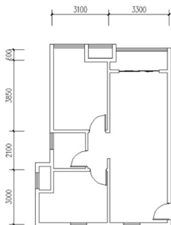
图2 理想建筑模型平面示意图
